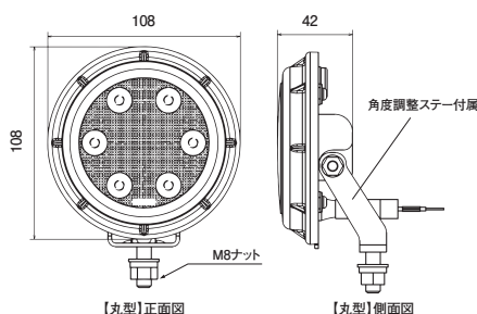
【丸型】正面図
