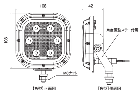
【角型】正面図
